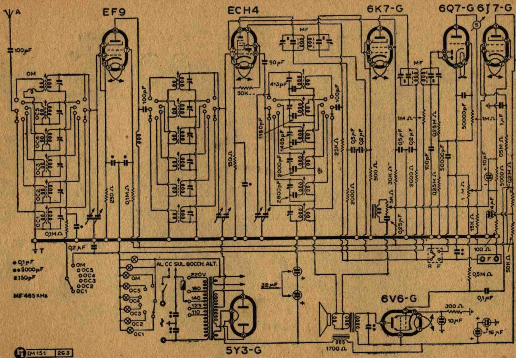
Lo schema elettrico del Mod. 716
